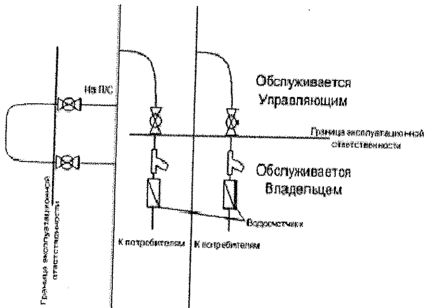
Трубопровод ГВС Трубопровод ХВС
